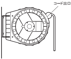
図 3. 壁面への取付け方法
