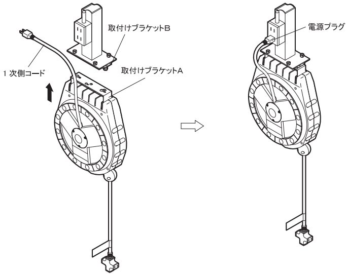
図 4. リールの取付け方法
