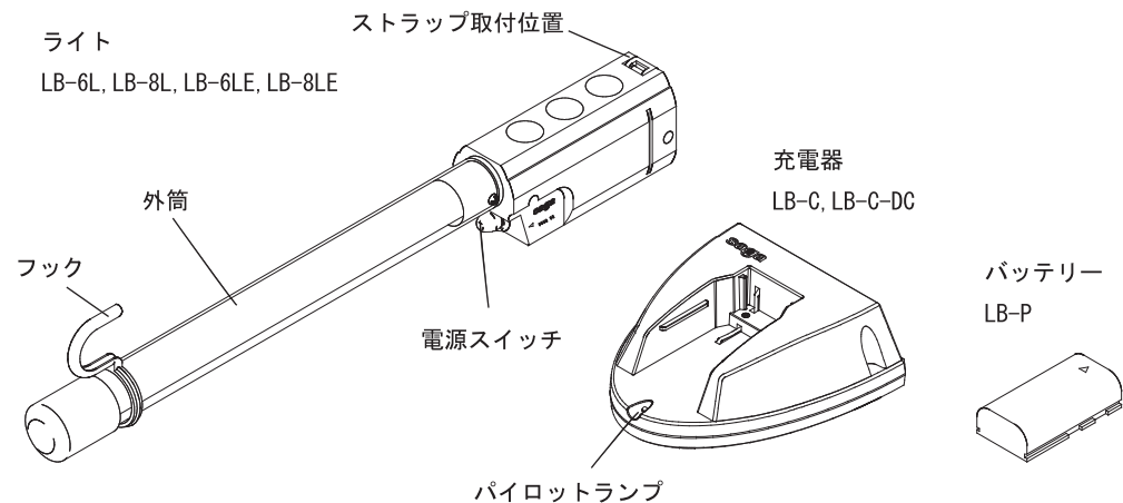
図1. セット型式（ライト+充電器+バッテリー）：LB-6, LB-8, LB-6D, LB-8D, LB-6E, LB-8E, LB-6ED, LB-8ED
