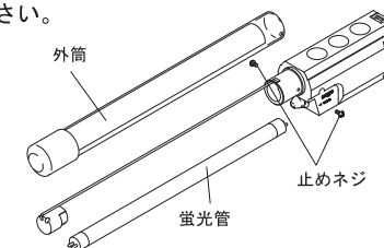
図3. 蛍光管の交換方法
