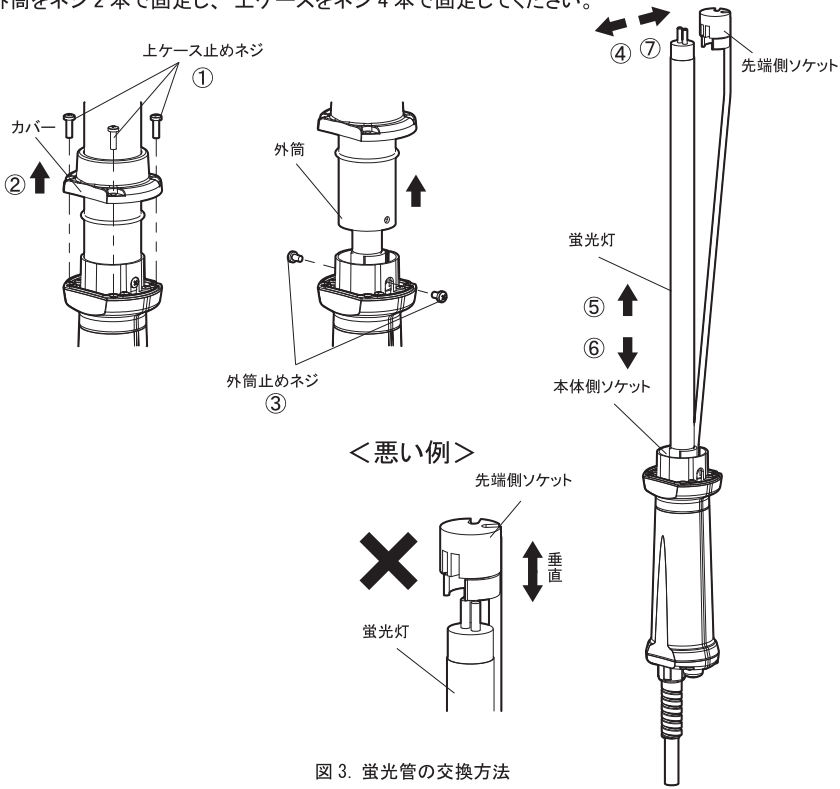
図 3. 蛍光管の交換方法
